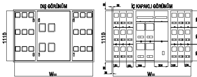
ÇP 3518 VE 3530 SERİSİ ÜÇ SIRA LI MONAFAZE SAYAÇ MODELİ Kompak, Bara, Zil Trafosu, Merdiven Otomatığı yeri mevcut + 4 Adet Trifaze
