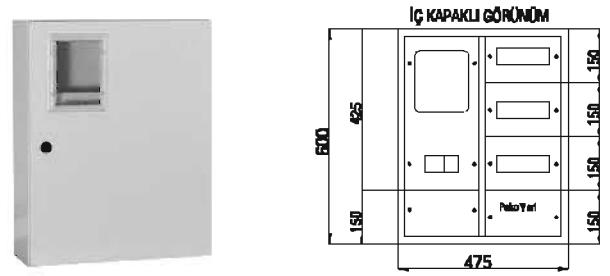
SIVA ÜSTÜ TRİFAZE DAĞITIM ve SAYAÇ PANOSU 1 Trifaze Sayaç 7 + 27 Ad. Sigorta + Pako Çıkışı
