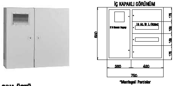
SİVA ÜSTÜ SAYAÇ + DAĞITIM PANOSU x 5 Kombi Sayaç, Dağıtım 32 Ad. Sigortalı
