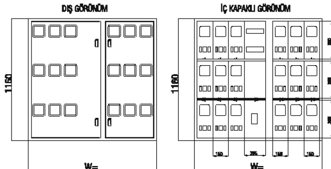
ÇP 3318S ve 3330S SERİSİ ÜÇ SIRA LI MONOFAZE SAYAÇ MODELİ Kompak, Bara, Zil Trafosu, Merdiven Otomatığı yeri mevcut
