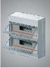
EUROBOX SERİSİ / HALOGEN FREE Sıva Üstü Sigorta Kutusu (IP 55) Gri RAL 7035
