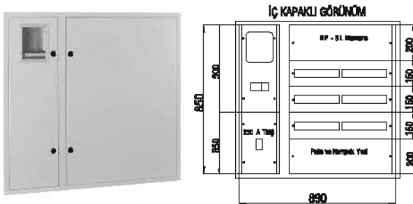
SIVA ALTI TRİFAZE DAĞITIM ve SAYAÇ PANOSU 1 Trifaze Sayaç 7 + 78 Ad. Sigorta + 250 A TMS. Çıkışı
