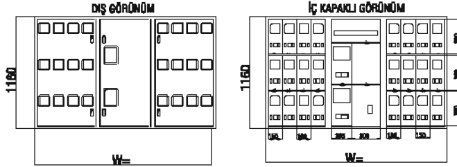
ÇP 3418S VE 3430S SERİSİ ÜÇ SIRALI MONAFAZE SAYAÇ MODELİ Kompak, Bara, Zil Trafosu, Merdiven Otomatığı yeri mevcut + 2 Adet Trifaze
