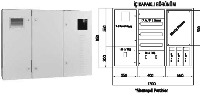
SİVA ÜSTÜ SAYAÇ + DAĞITIM + KOMPANZASYON PANOSU x 5 Kombi Sayaç, 51 Ad. Sigortalı 8 Kademe Kompanzasyon
