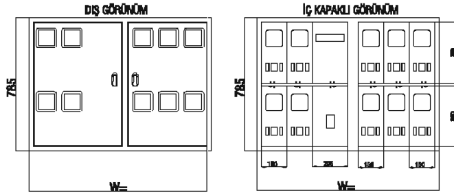
ÇP 304S ve 320S SERİSİ İKİ SIRA LI MONOFAZE SAYAÇ MODELİ Kompak, Bara, Zil Trafosu, Merdiven Otomatığı yeri mevcut
