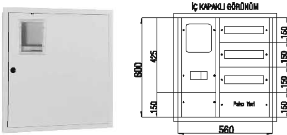
SIVA ALTI TRİFAZE DAĞITIM ve SAYAÇ PANOSU 1 Trifaze Sayaç 7 + 39 Ad. Sigorta + Pako Çıkışı
