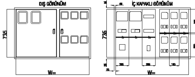
ÇP 404 VE 420 SERİSİ İKİ SIRA LI MONAFAZE SAYAÇ MODELİ Kompak, Bara, Zil Trafosu, Merdiven Otomatığı yeri mevcut + 2 Adet Trifaze
