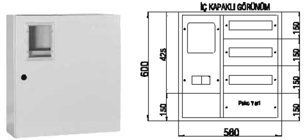
SIVA ÜSTÜ TRİFAZE DAĞITIM ve SAYAÇ PANOSU 1 Trifaze Sayaç 7 + 39 Ad. Sigorta + Pako Çıkışı
