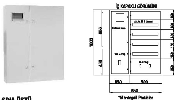
SİVA ÜSTÜ SAYAÇ + DAĞITIM PANOSU x 5 Kombi Sayaç, Dağıtım 84 Ad. Sigortalı
