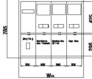
İÇ KAPAKLI GÖRÜNÜM
