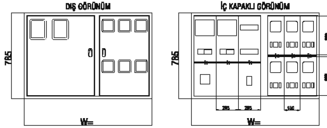
ÇP 404S VE 420S SERİSİ İKİ SIRALI MONAFAZE SAYAÇ MODELİ Kompak, Bara, Zil Trafosu, Merdiven Otomatığı yeri mevcut + 2 Adet Trifaze
