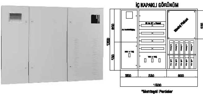
SİVA ÜSTÜ SAYAÇ + DAĞITIM + KOMPANZASYON PANOSU x 5 Kombi Sayaç, 96 Ad. Sigortalı 12 Kademe Kompanzasyon
