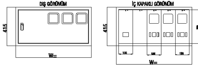
ÇP 302S ve 303S SERİSİ TEK SIRA LI MONOFAZE SAYAÇ MODELİ Kompak, Bara, Zil Trafosu, Merdiven Otomatığı yeri mevcut
