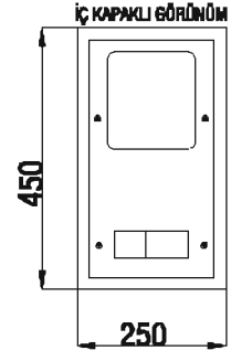
SIVA ÜSTÜ TRİFAZE DAĞITIM ve SAYAÇ PANOSU 1 Trifaze Sayaç Kolon Sigorta Çıkışlı
