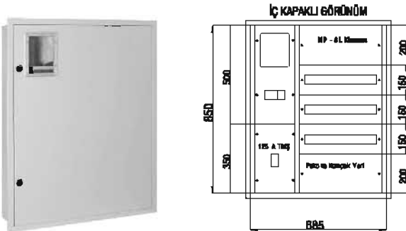
SIVA ALTI TRİFAZE DAĞITIM ve SAYAÇ PANOSU 1 Trifaze Sayaç 7 + 60 Ad. Sigorta + 125 A TMS. Çıkışı
