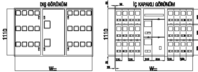
ÇP 3418 VE 3430 SERİSİ ÜÇ SIRA LI MONAFAZE SAYAÇ MODELİ Kompak, Bara, Zil Trafosu, Merdiven Otomatığı yeri mevcut + 2 Adet Trifaze
