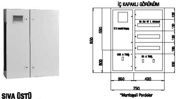
SİVA ÜSTÜ SAYAÇ + DAĞITIM PANOSU x 5 Kombi Sayaç, Dağıtım 48 Ad. Sigortalı
