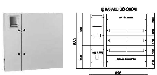
SIVA ÜSTÜ TRİFAZE DAĞITIM ve SAYAÇ PANOSU 1 Trifaze Sayaç 7 + 78 Ad. Sigorta + 250 A TMS. Çıkışı
