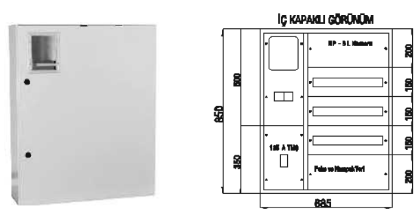
SIVA ÜSTÜ TRİFAZE DAĞITIM ve SAYAÇ PANOSU 1 Trifaze Sayaç 7 + 60 Ad. Sigorta + 125 A TMS. Çıkışı
