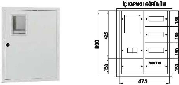
SIVA ALTI TRİFAZE DAĞITIM ve SAYAÇ PANOSU 1 Trifaze Sayaç 7 + 27 Ad. Sigorta + Pako Çıkışı
