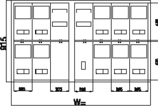
İÇ KAPAKLI GÖRÜNÜM
