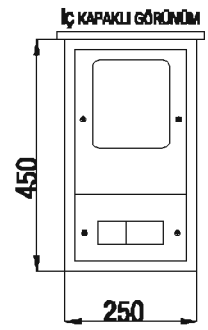
SIVA ÜSTÜ TRİFAZE DAĞITIM ve SAYAÇ PANOSU 1 Trifaze Sayaç Kolon Sigorta Çıkışlı Çablı
