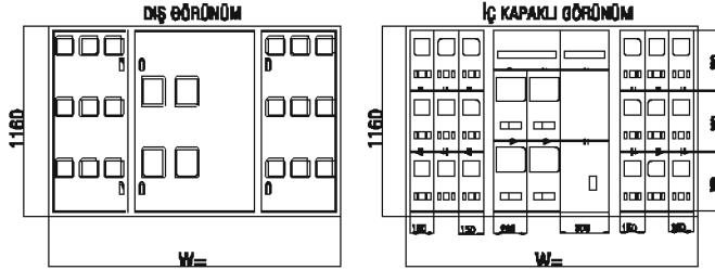
ÇP 3518S VE 3530S SERİSİ ÜÇ SIRALI MONAFAZE SAYAÇ MODELİ Kompak, Bara, Zil Trafosu, Merdiven Otomatığı yeri mevcut + 4 Adet Trifaze
