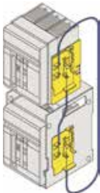
2'li dikey mekanik kilit
