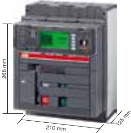
X1B 1250A 3p F F PR332/P-LI
